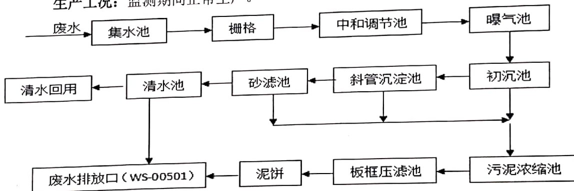
图 1 废水处理流程图
